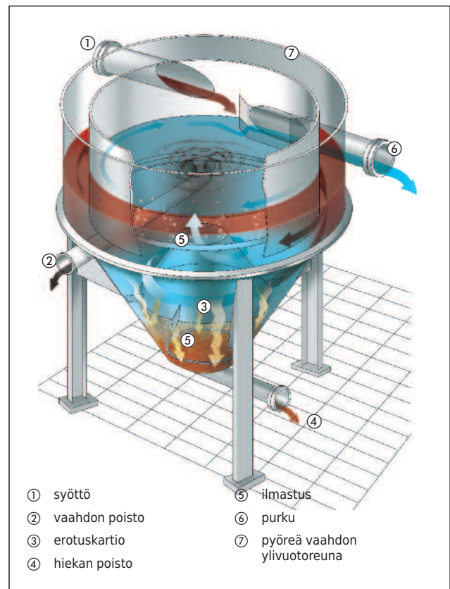
HUBER Pyöreän hiekanerotin HRSF, virtauskaavio
